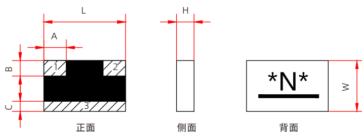
G和W0封装形式产品外形图
