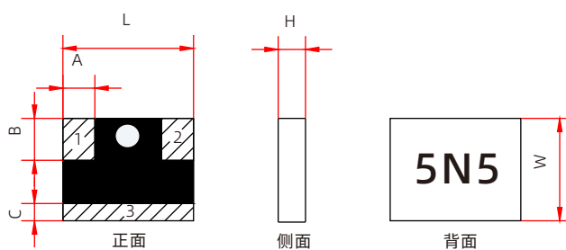
G和W0封装形式产品外形图
