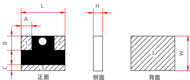
WB1封装形式产品外形图
