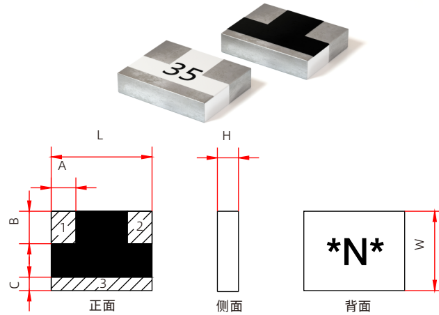
G和W0封装形式产品外形图
